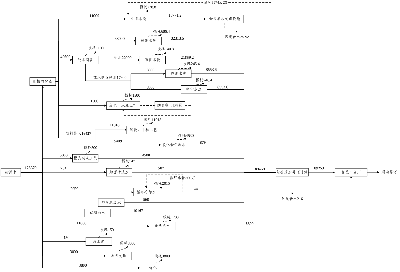
图 4.2.2-5 本项目水平衡图 (t/a)
