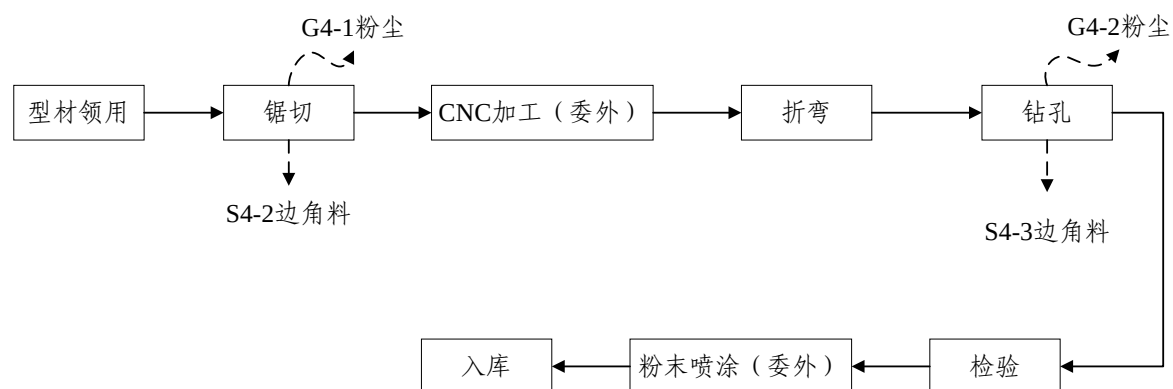
图 4.2.2-5 平衡车零配件组装工艺流程及产排污节点图
