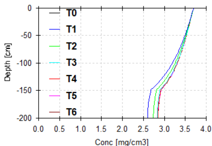
图 6.6.3-6 事故发生后土壤层不同深度总镍浓度随时间变化图 (N1=0.2m、N2=0.5m、N3=1.0m、N4=1.5m、N5=2.0m)
