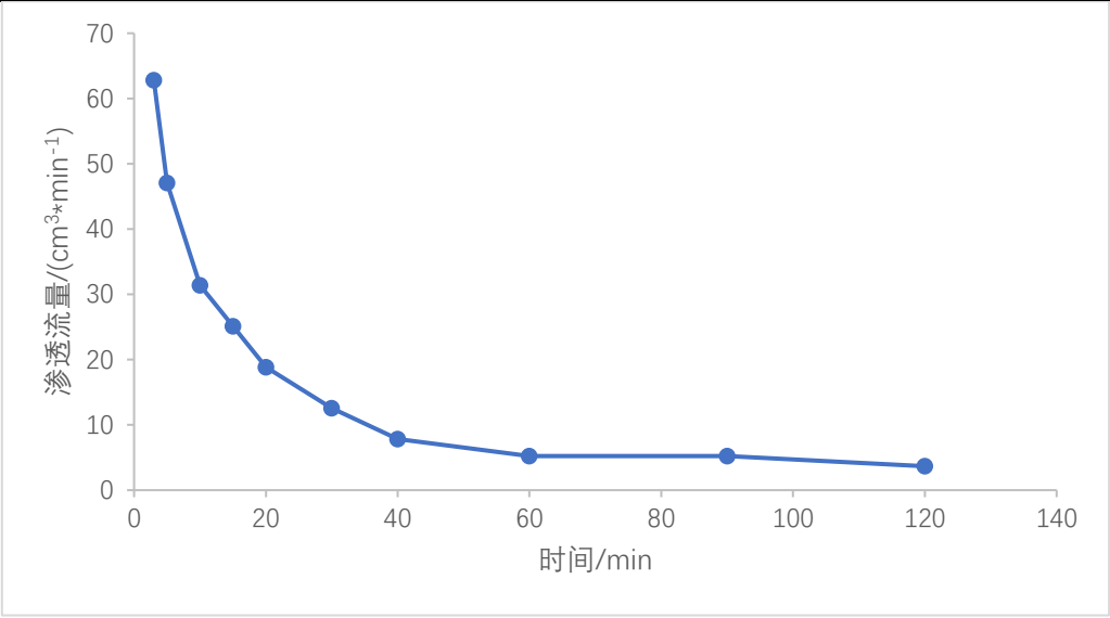
图 5.3.6-3 渗水试验渗透流量历时曲线
