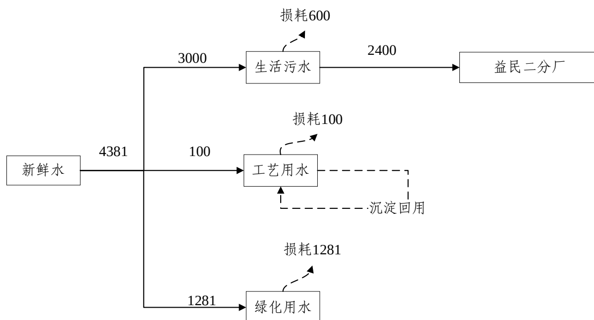
图 3.2.1-1 现有项目水平衡图
