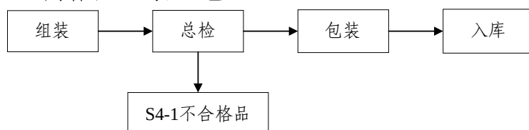
图 4.2.2-4 多功能登高器具组装工艺流程及产排污节点图
