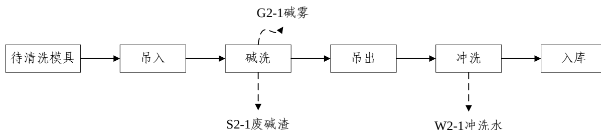
图 4.2.2-2 模具碱洗生产工艺流程及产排污节点图
