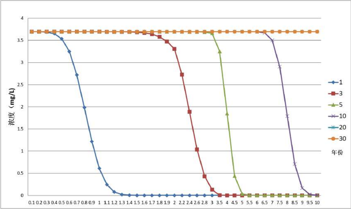
图 6.5.2-1 非正常排放总镍浓度变化图
