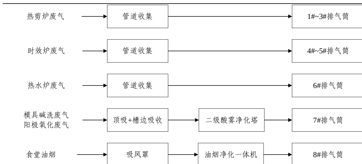
图 7.2.1-1 项目废气处理线路图
