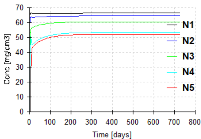
图 6.6.3-4 事故发生后土壤层不同深度石油类浓度随时间变化图
