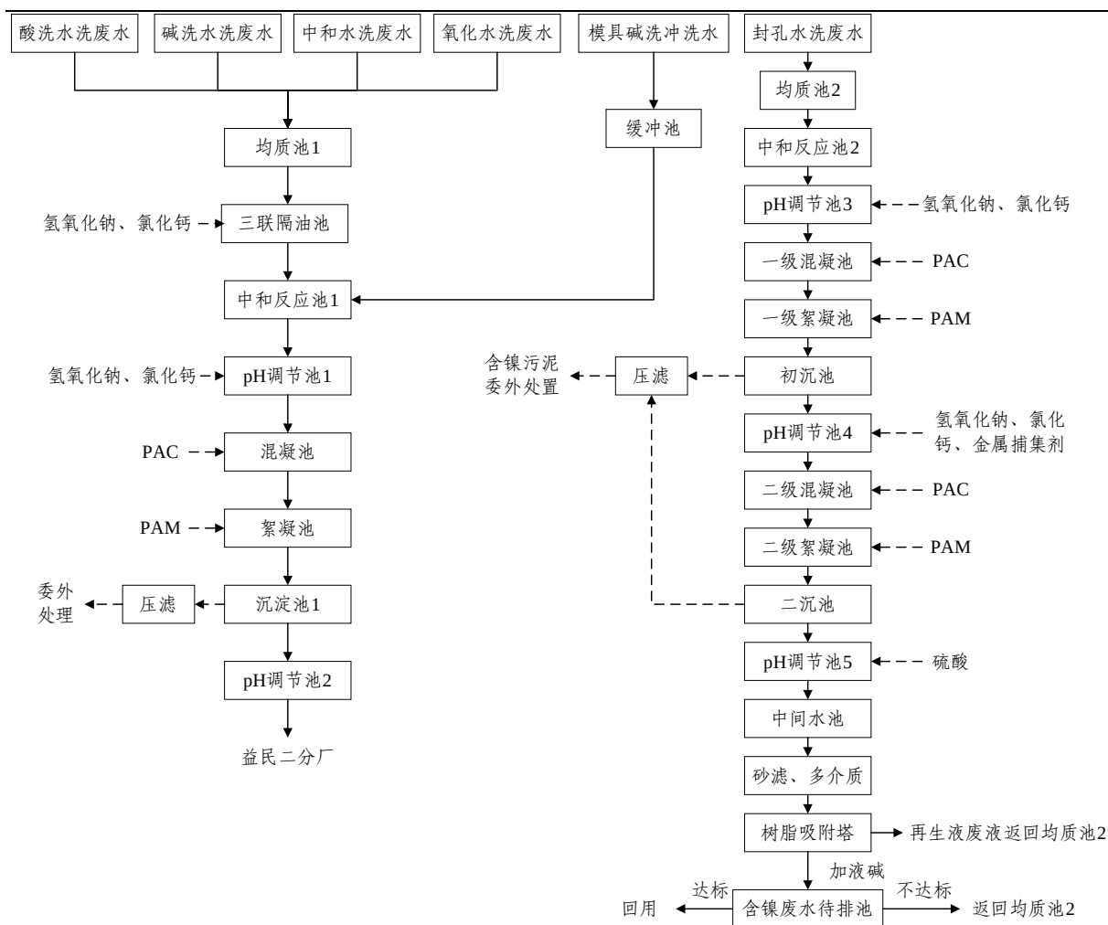
图 7.2.2-1 本项目废水处理工艺流程图
