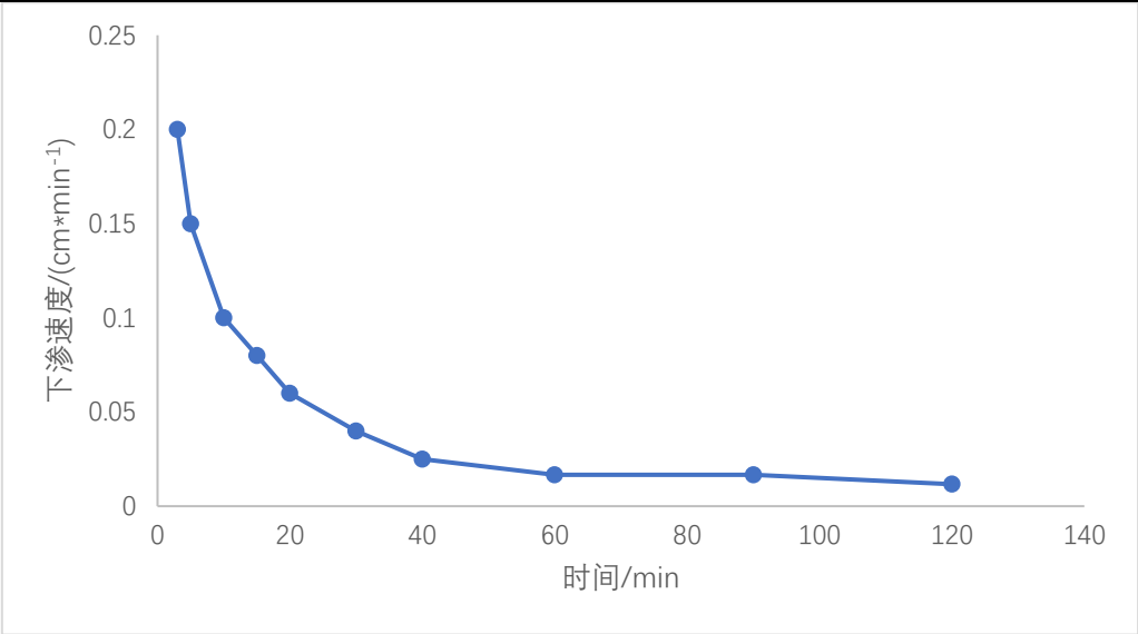
图 5.3.6-4 渗水试验下渗速度历时曲线
