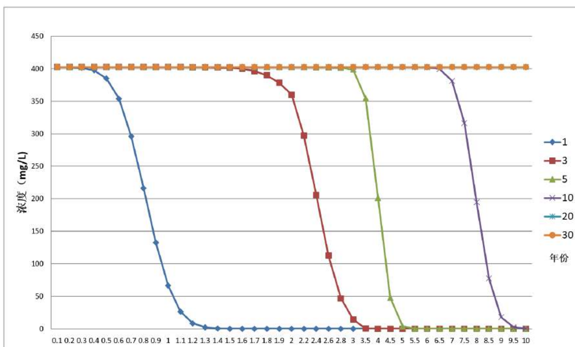
图 6.5.2-2 非正常排放 COD 浓度变化图
