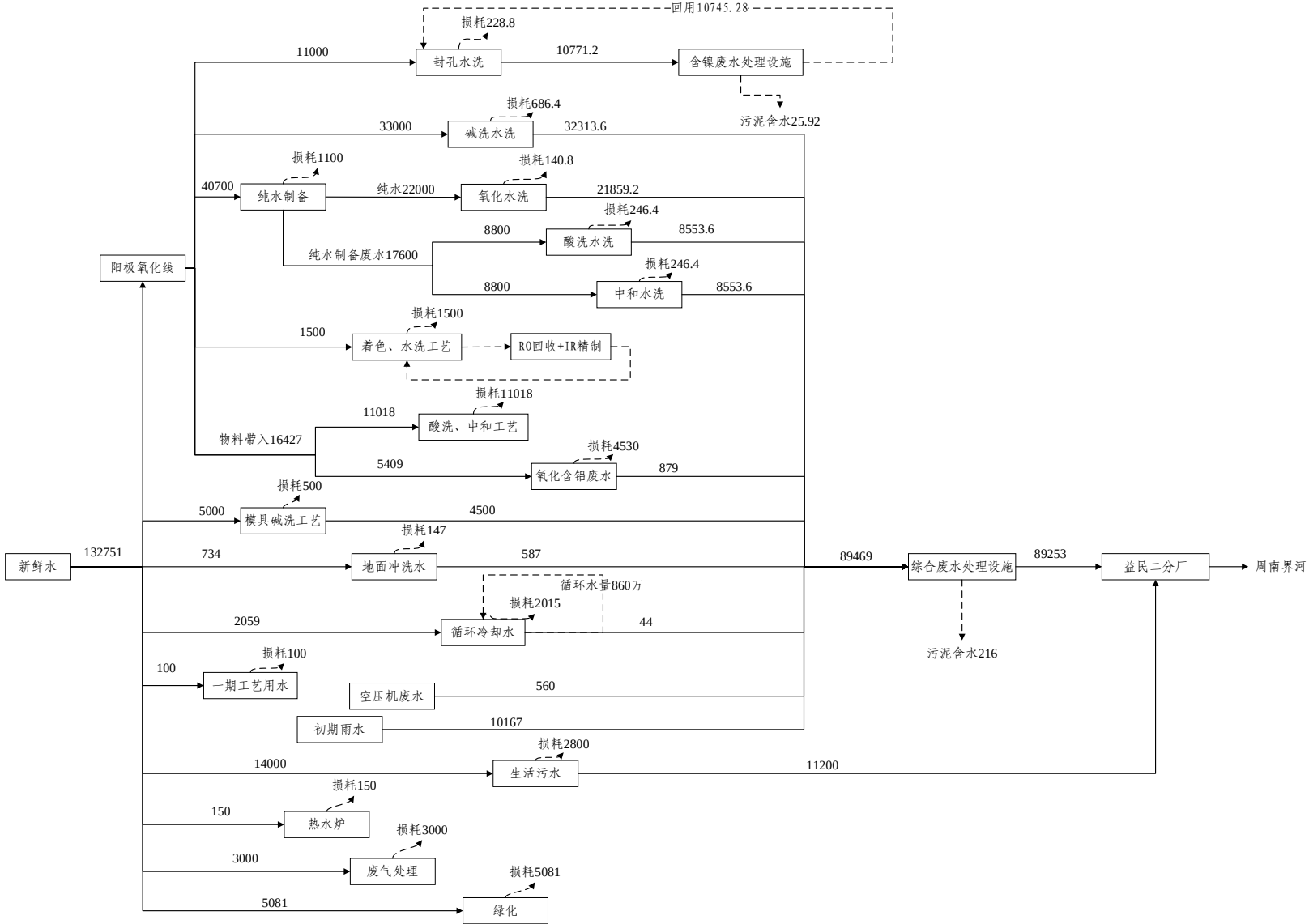
图 4.2.2-6 本项目建成后全厂水平衡图
